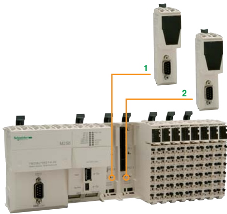
1 Модуль связи TM5 PCRS – последовательный интерфейс Modbus/ASCII; 2 Модуль связи TM5 PCDPS: линия подключения к ведомому устройству Profibus DP.
