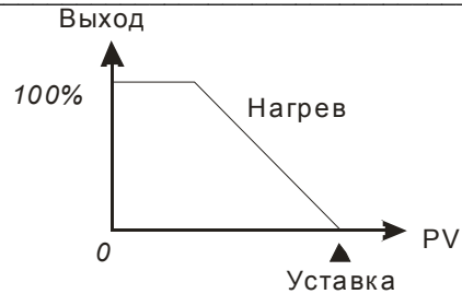
Рис 3: ПИД-регулирование, управление охлаждением
