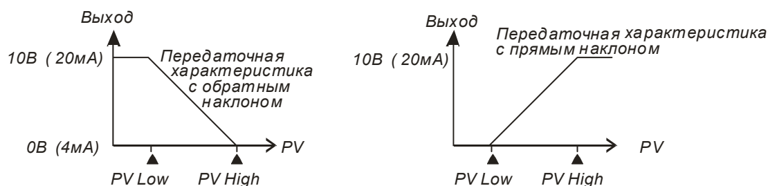
Рис 7: Пропорциональный выход
